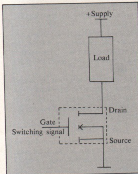
Figure VII: A VMOS FET
